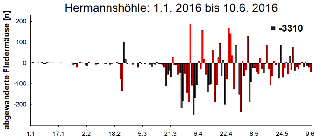
Abb.4. Abwanderungsverlauf überwinternder Fledermäuse auf Basis bilanzierter Lichtschrankenregistrierungen.
