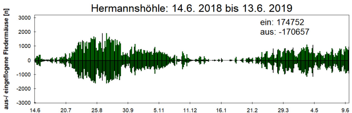
Abb.2. Fledermausaktivität auf Basis der Registrierungen der vier Lichtschranken.
