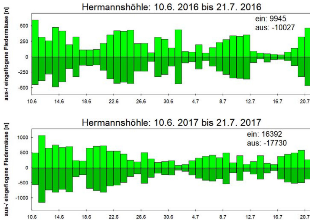
Abb.3. Fledermausaktivität an den vier Lichtschranken im Zeitraum vom 10. Juni bis 21. Juli in den Jahren 2016 und 2017.
